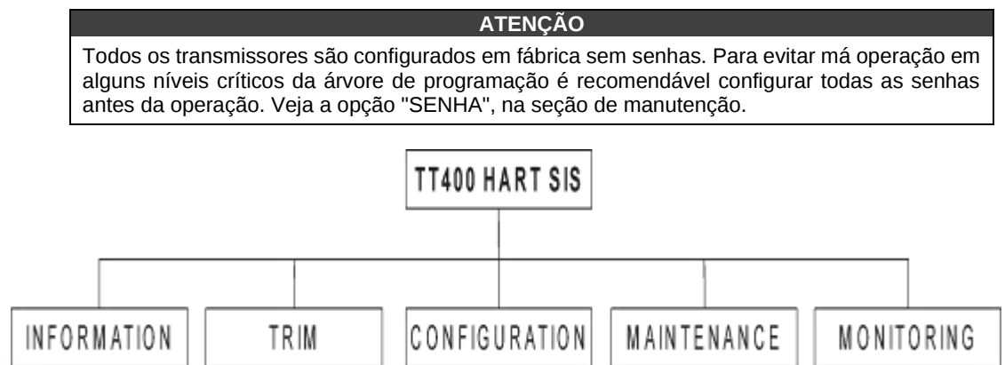
Figura 3.3 – Árvore do Configurador
