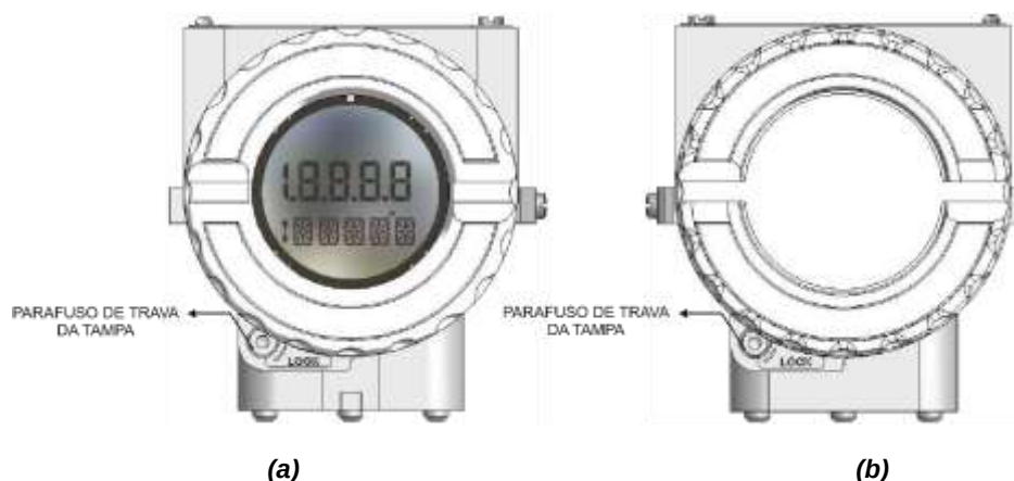
Figura 1.2 – (a) Trava da Tampa do Display (b) Parafuso da Trava dos Terminais
