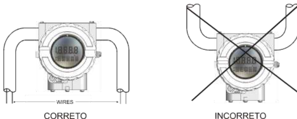
Figura 1.3 - Diagrama de Instalação do Eletroduto
