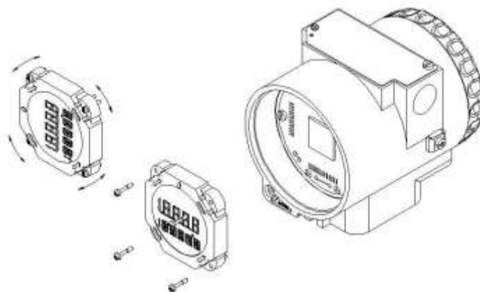
Figura 4.2 – Quatro Posições Possíveis do Display
