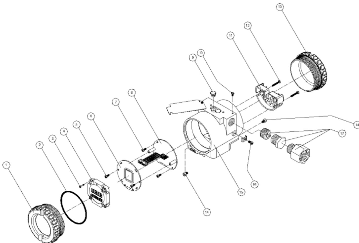
Figura 4.1 – Desenho Explodido
