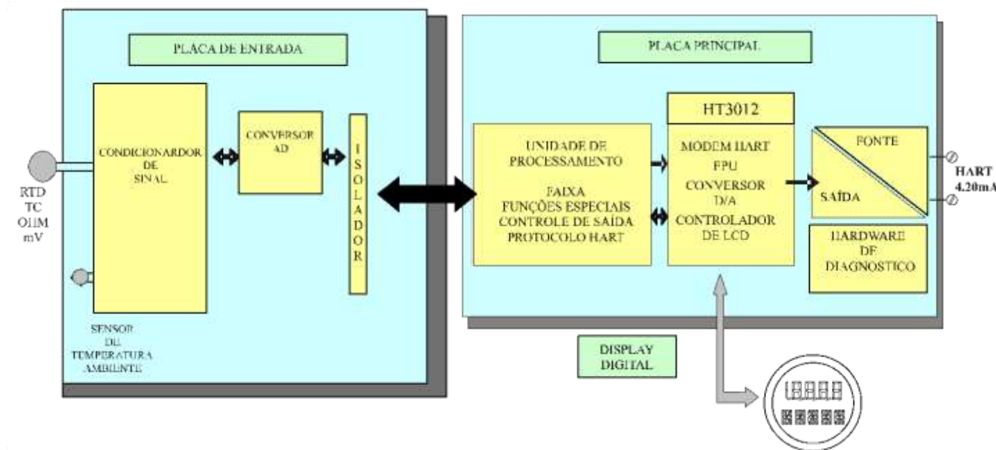
Figura 2.1 - Diagrama de Bloco do TT400 SIS
