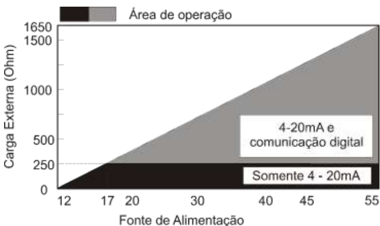
Figura 1.6 - Reta de Carga
