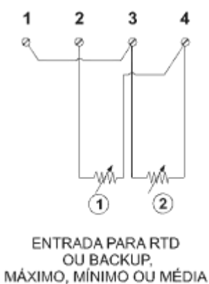
Figura 1.7 - Ligação do Sensor
