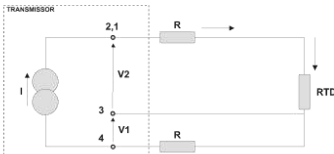
Figura 2.3 - Conexão a 3-Fios
