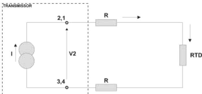
Figura 2.2 - Conexão a 2-Fios
