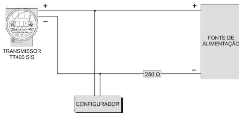
Figura 1.5 - Diagrama de Ligação do TT400 HART® SIS
