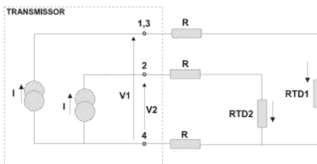
Figura 2.5 - Conexão Diferencial
