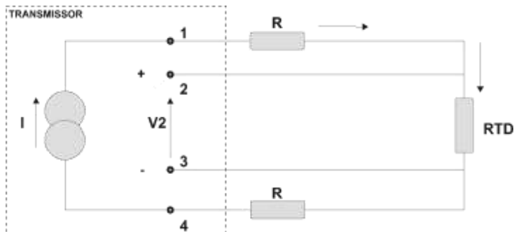
Figura 2.4 - Conexão a 4-Fios
