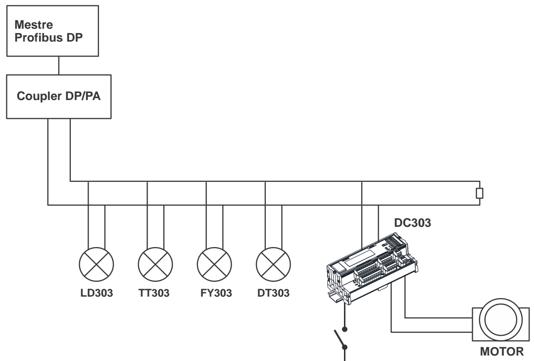
Figure 3.4 - Aplicação 2 - DC303
