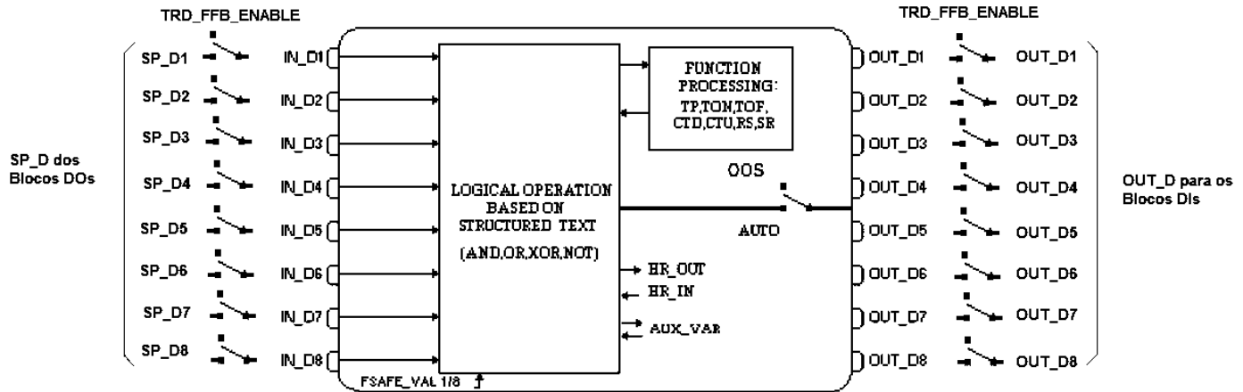
Figura 3.6 - Esquemático
