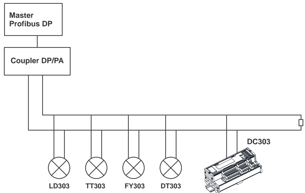
Figura 1.9 – DC303 e um Sistema Genérico Profibus
