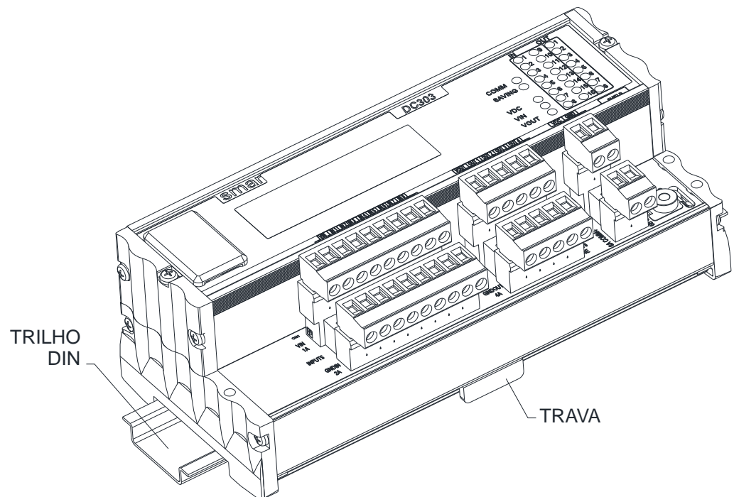
Figura 1.1- Montagem Mecânica
