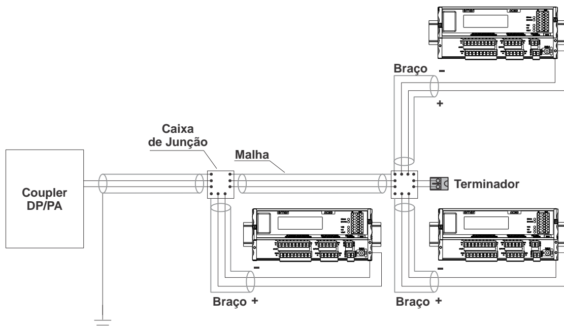
Figura 1.7 - Topologia Barramento
