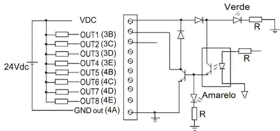
Figura 1.6 – Exemplo de conexões de saída
