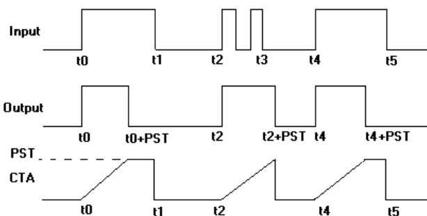
Figura 3.7 - Função Timer Pulse – diagramas de tempo
