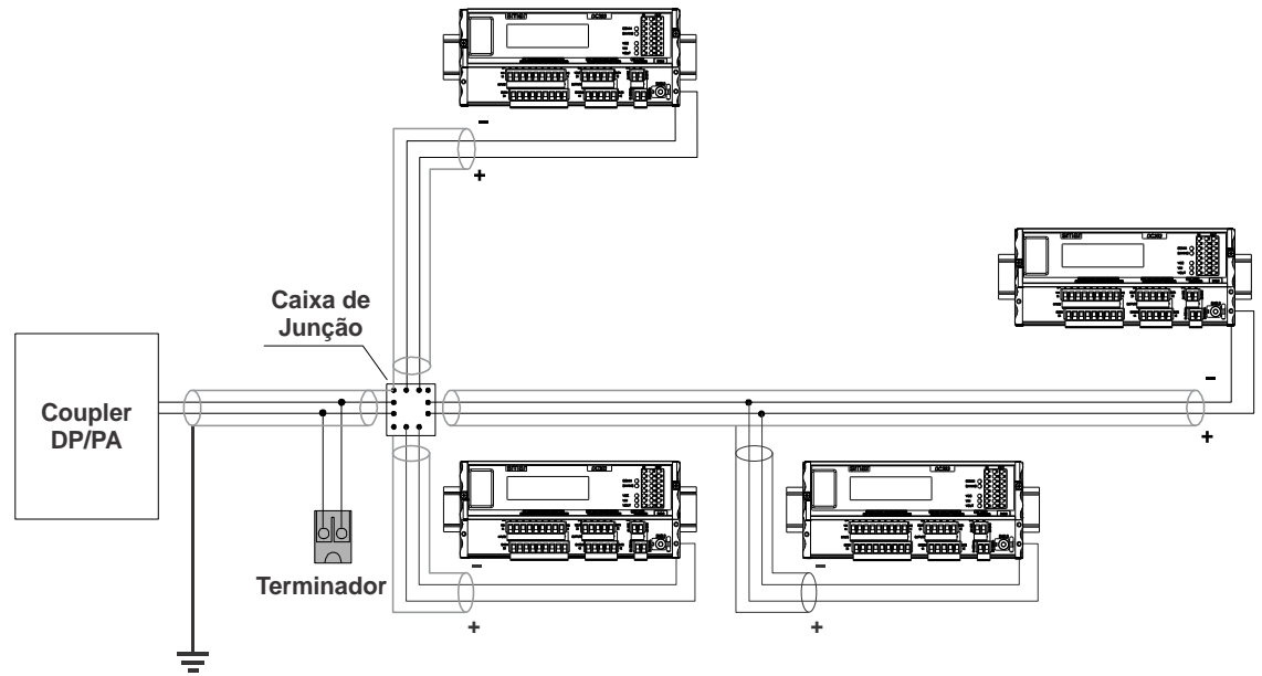
Figura 1.8 – Topologia Árvore
