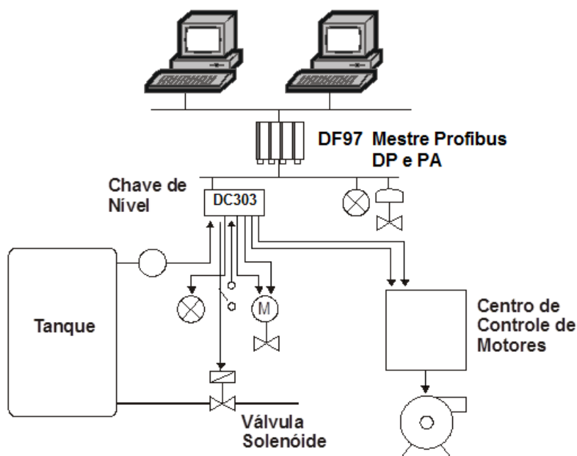
Figure 3.5 - Aplicação 5 - DC303
