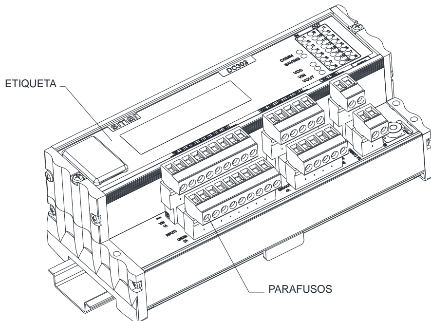
Figura 1.3 – Bloco de conexões
