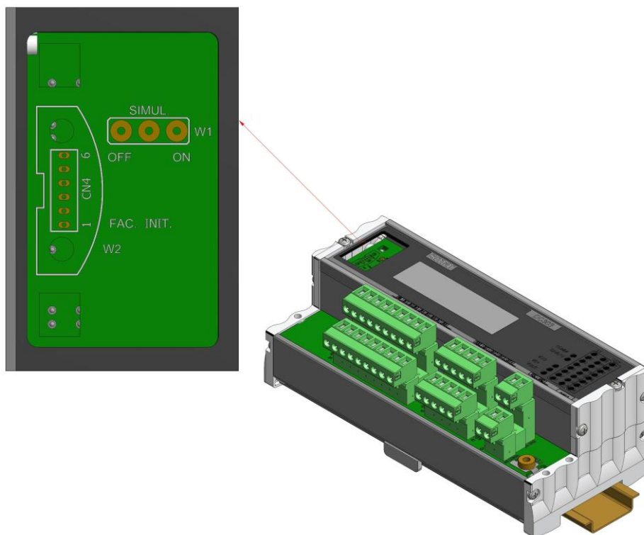
Figura 3.15 - Vista superior do DC303 com detalhe do Simulation Jumper habilitado na posição ON.
