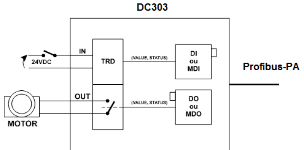
Figure 3.3 - Aplicação 1- DC303
