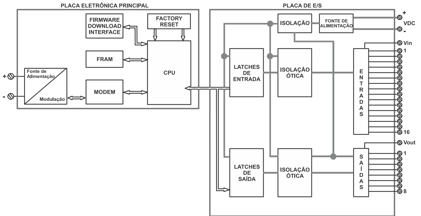
Figura 2.1 – Diagrama de Blocos DC303
