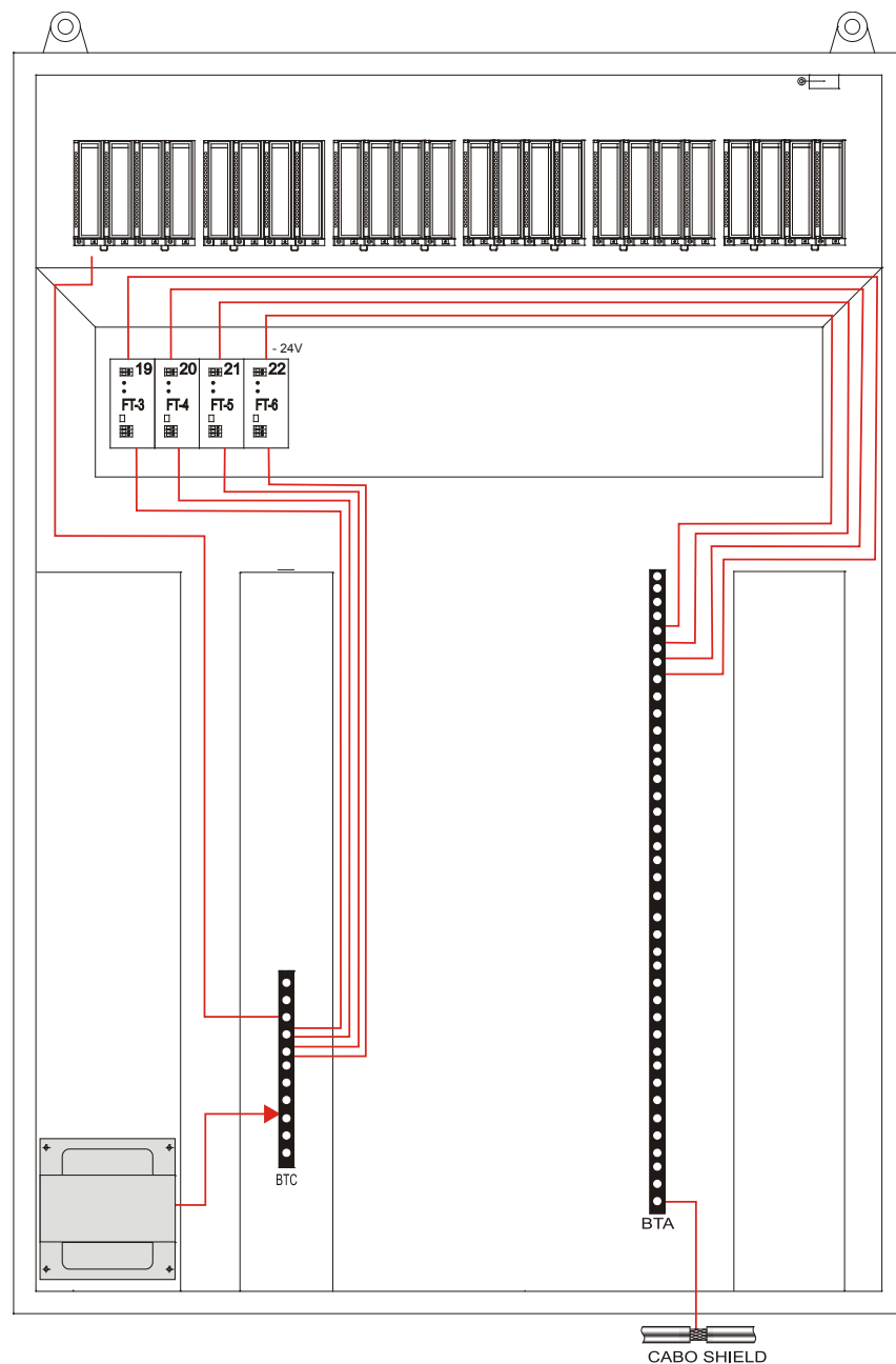
Figura 9.5 – Conexões para a Barra de Terra Analógico e para a Barra de Terra de Carcaça
