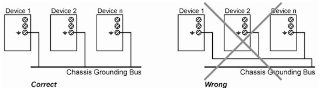
Figura 9.2 – Conexão Correta ao Barramento de Aterramento dos Chassis
