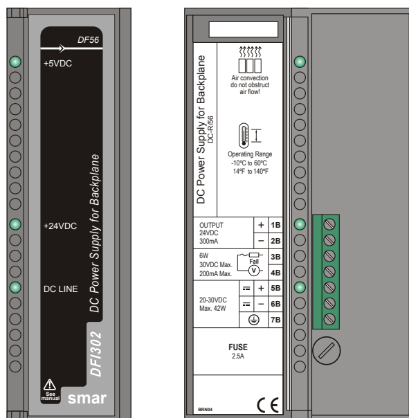
Figura 5. 2 – Módulo Fonte de Alimentação DC: DF56
