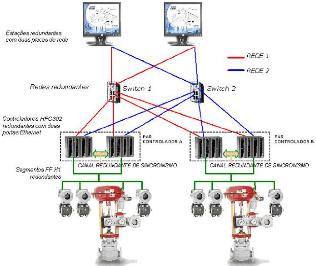
Figura 14. 1 – Arquitetura Redundante
