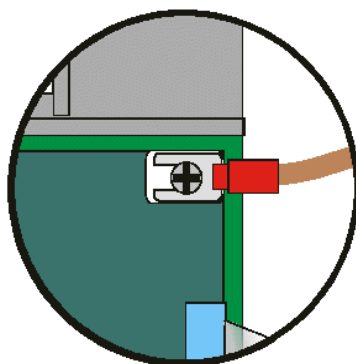
Figura 3. 26 - Detalhe de conexão do cabo de terra
