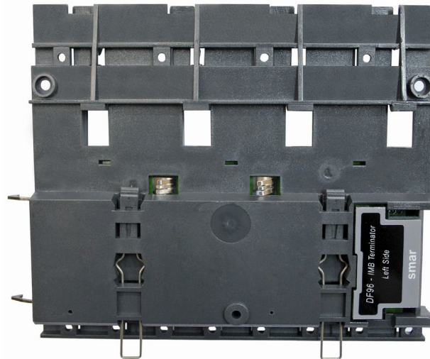
Figura 3. 13 – Terminador DF96 instalado no rack DF93
