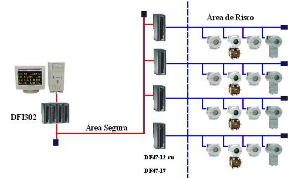
Figura 5. 13 – Instalação do DF47
