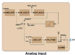
Analog Input
