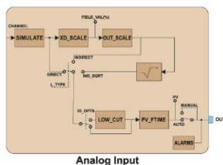
Analog Input
